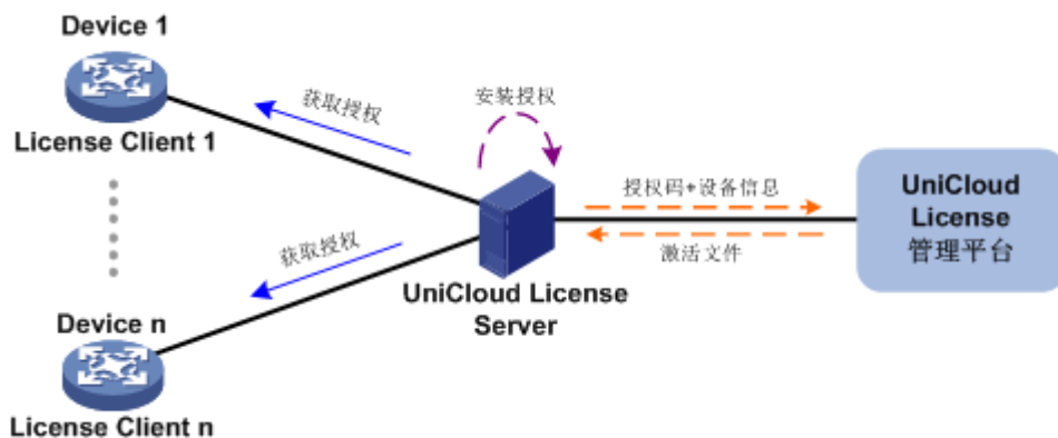
图1-1 远程授权示意图
