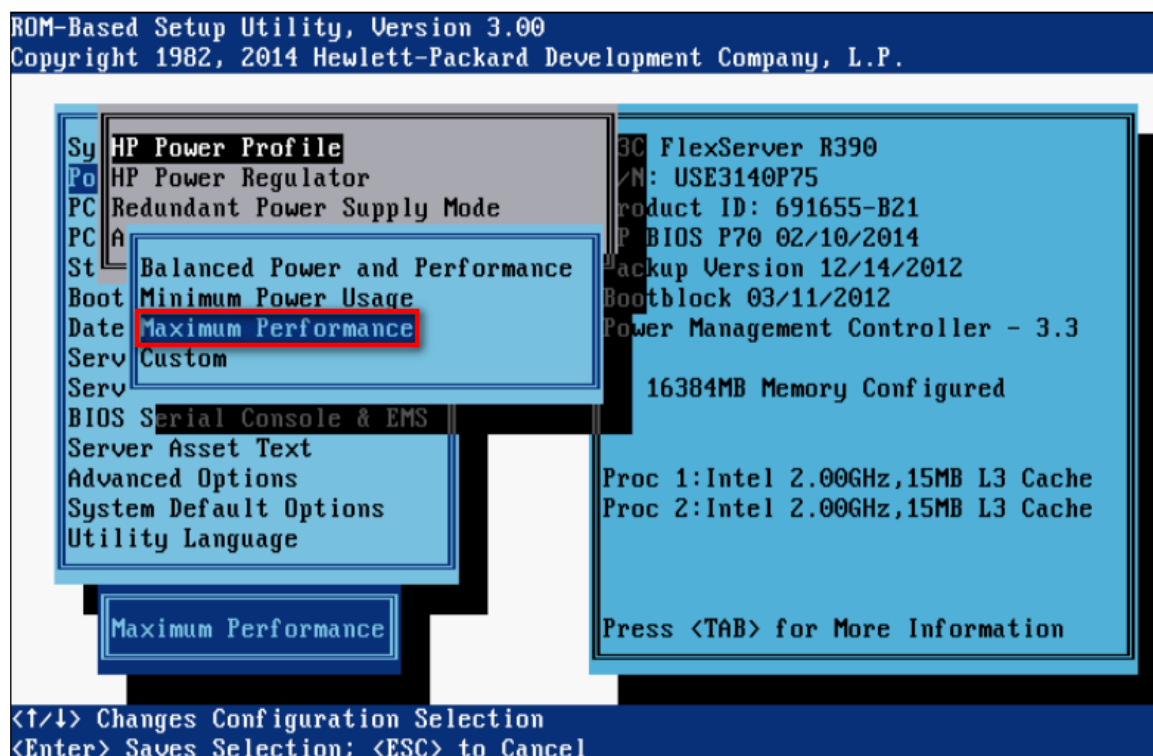
图4-1 配置电源
