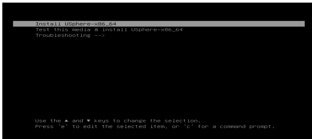
图4-4 启动安装
