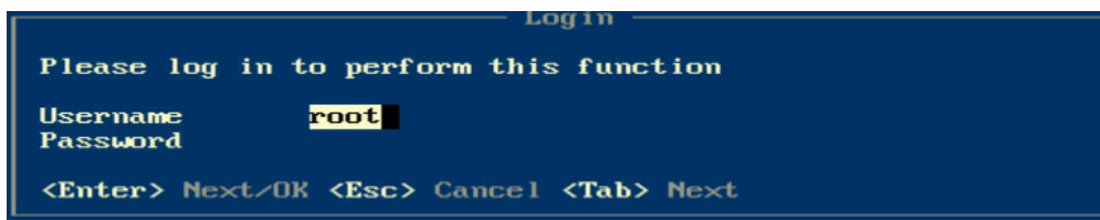
图4-26 Login 对话框
