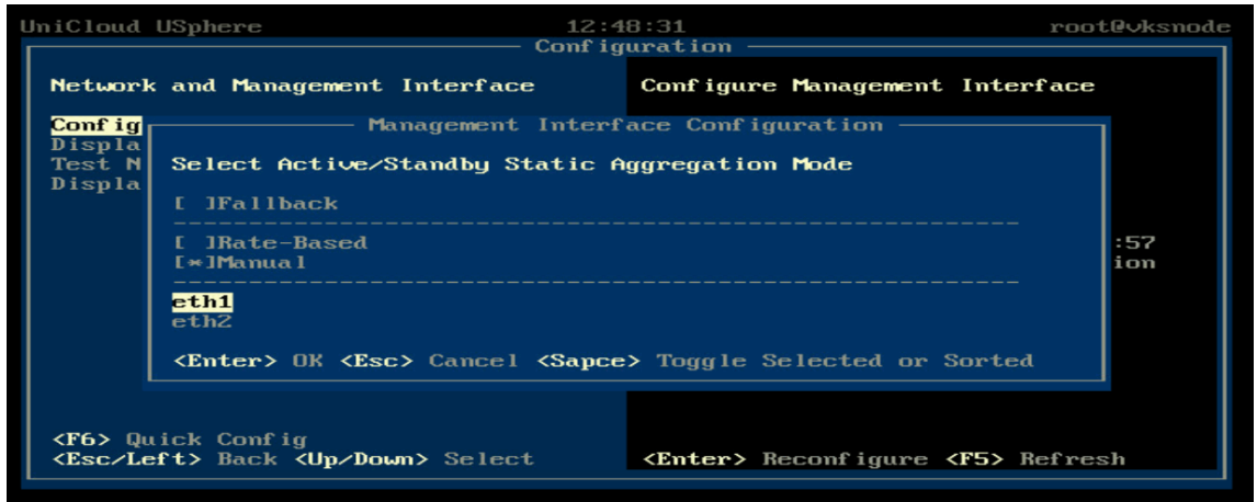
图4-33 指定优先级
