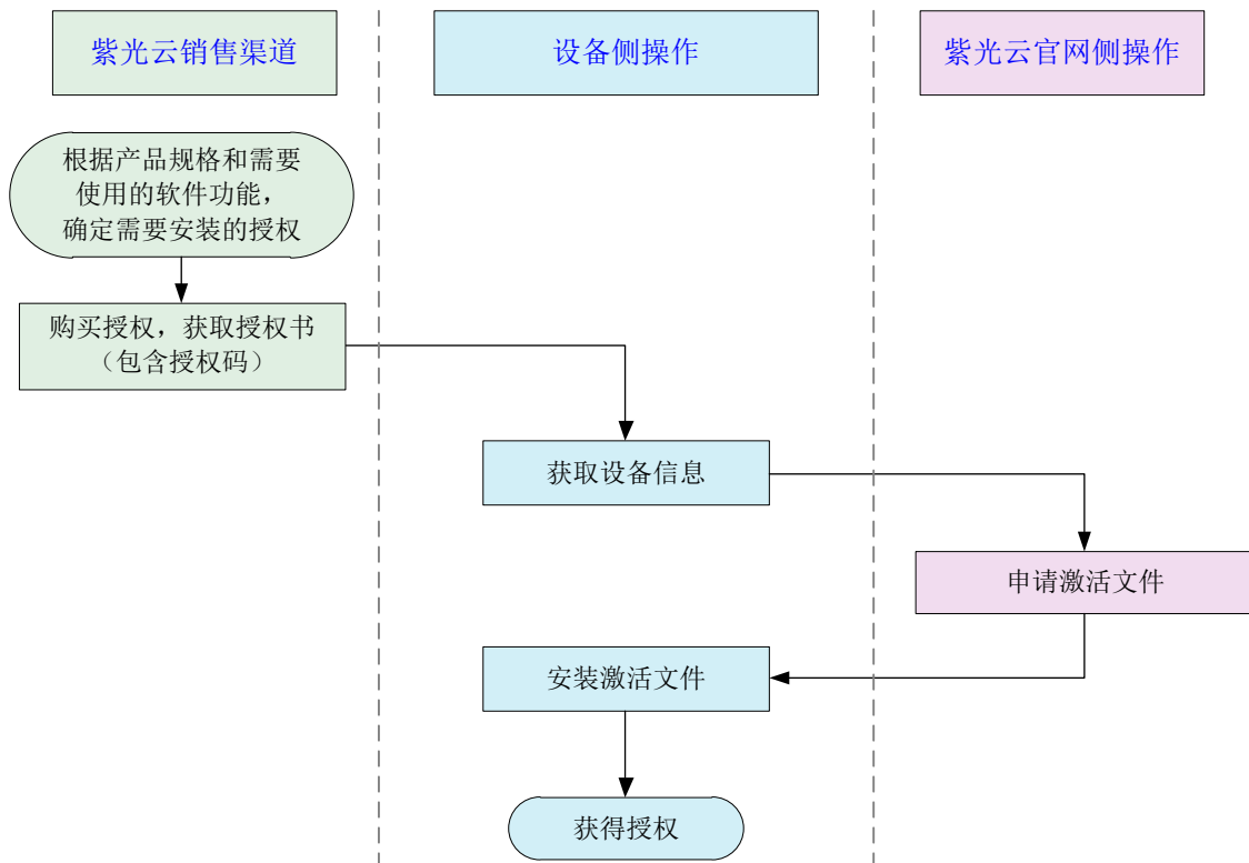
图2-3 License 本地授权通用安装流程图
