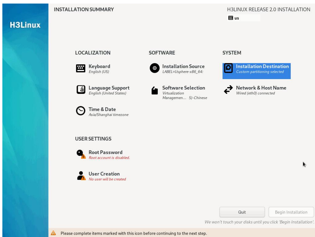
图 4-19 系统安装页面
