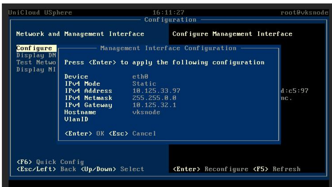
图 4-30 设置静态 IP 页面
