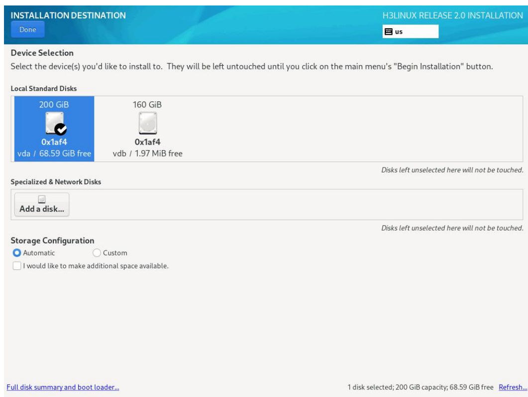
图 4-12 选择系统盘-自动分区
