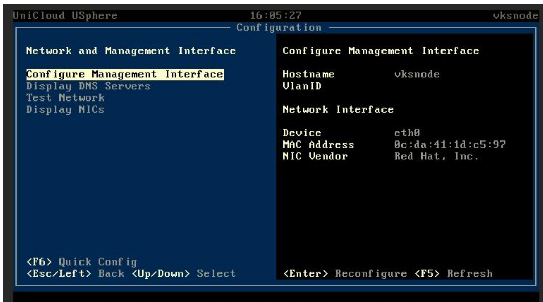
图 4-27 Configure Management Interface 页面
