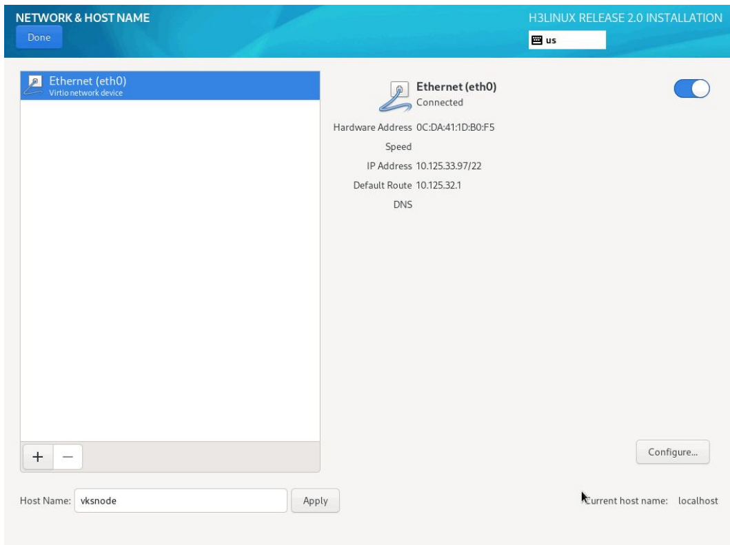
图 4-8 设置主机名，打开网卡
