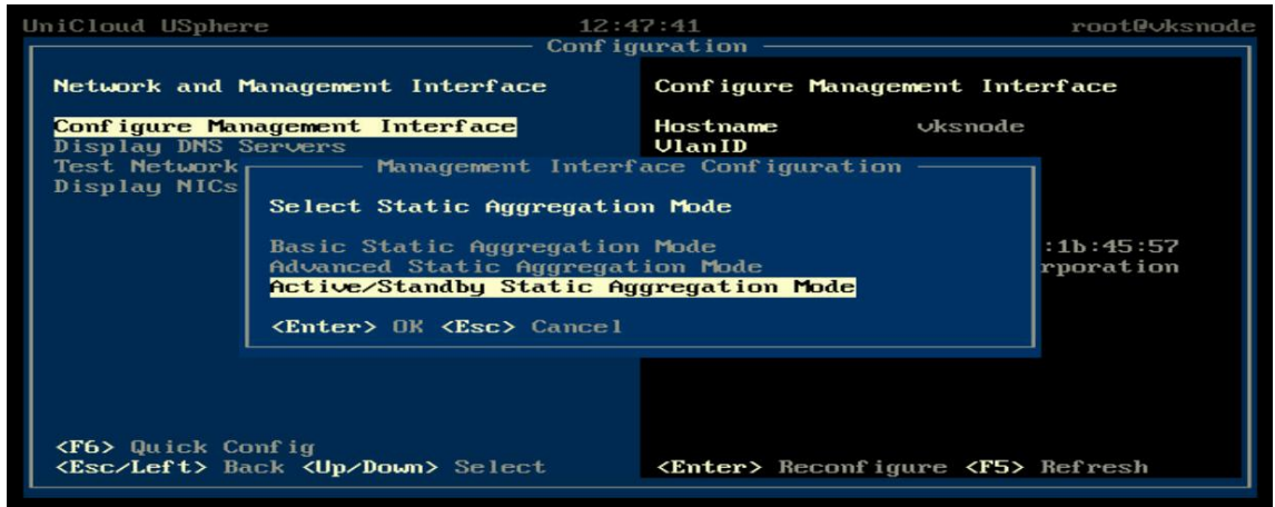
图 4-34 配置负载分担
