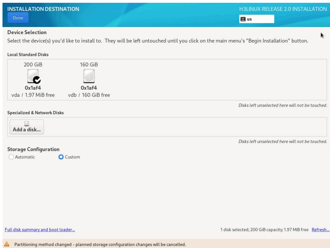
图 4-14 选择系统盘-手动分区
