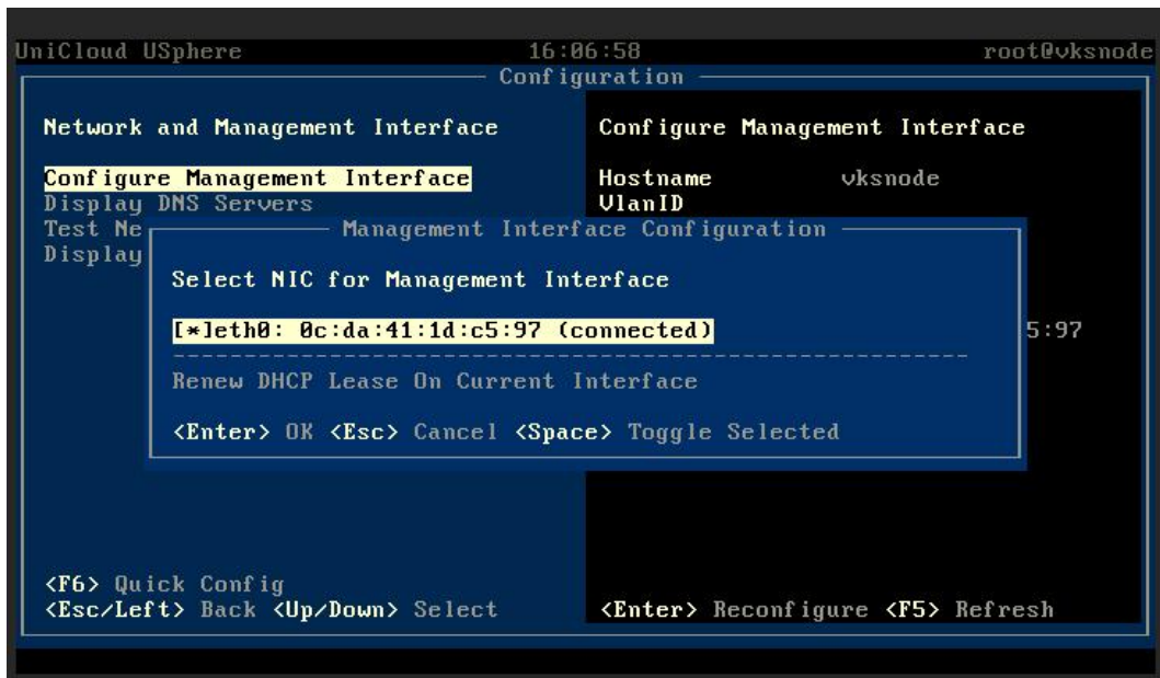
图 4-29 选择管理网网卡页面
