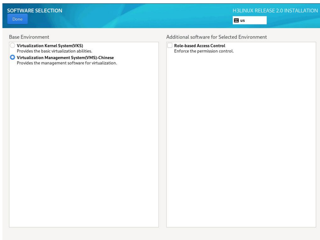
图 4-21 根据服务器类型选择安装 Usphere 组件
