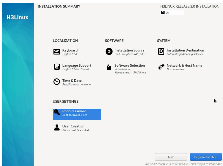
图 4-23 开始安装
