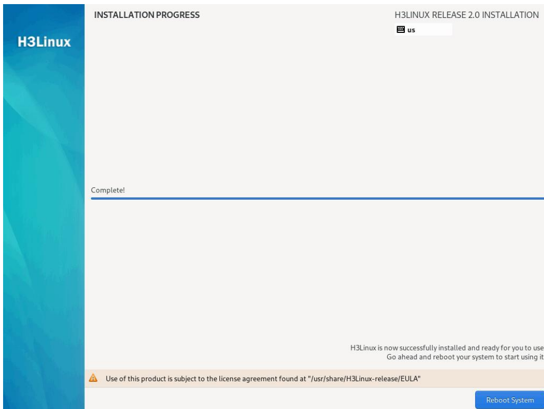
图 4-24 重启服务器
