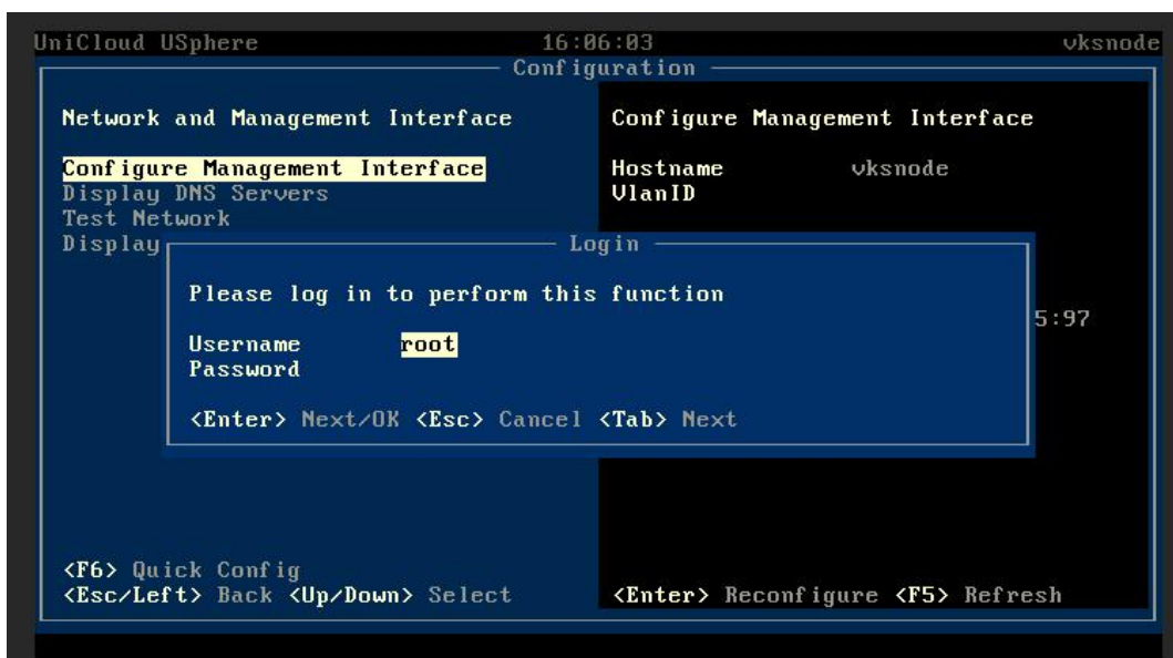
图 4-28 Login 对话框
