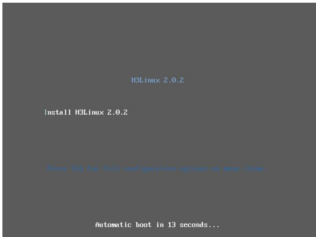
图 4-4 启动安装
