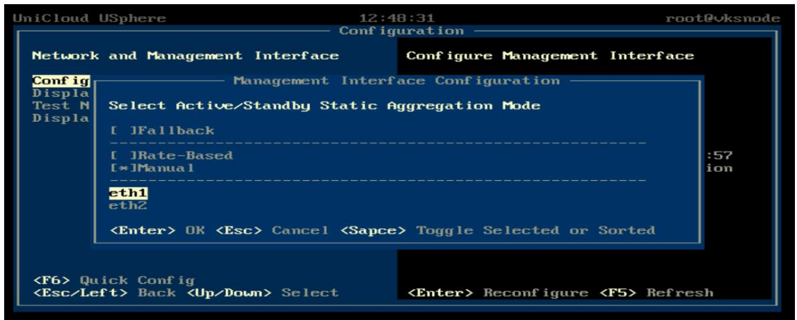
图 4-35 指定优先级
