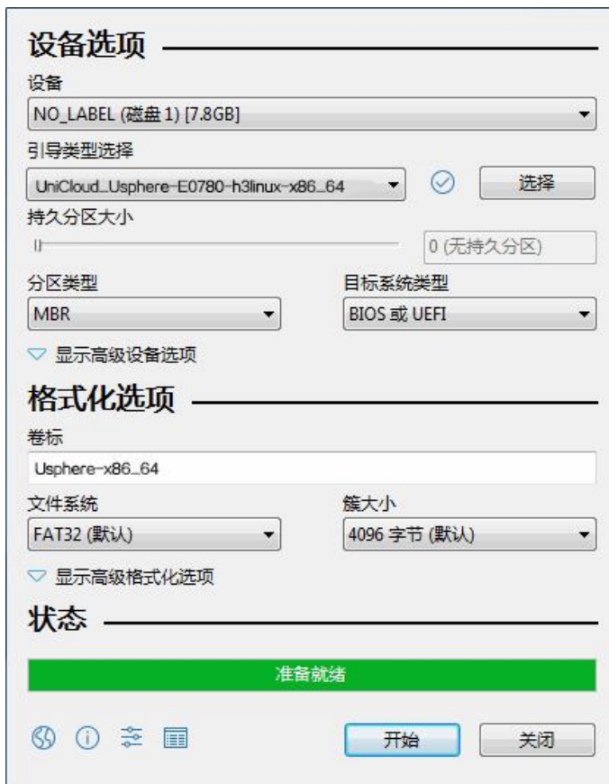
图 7-5 开始制作
