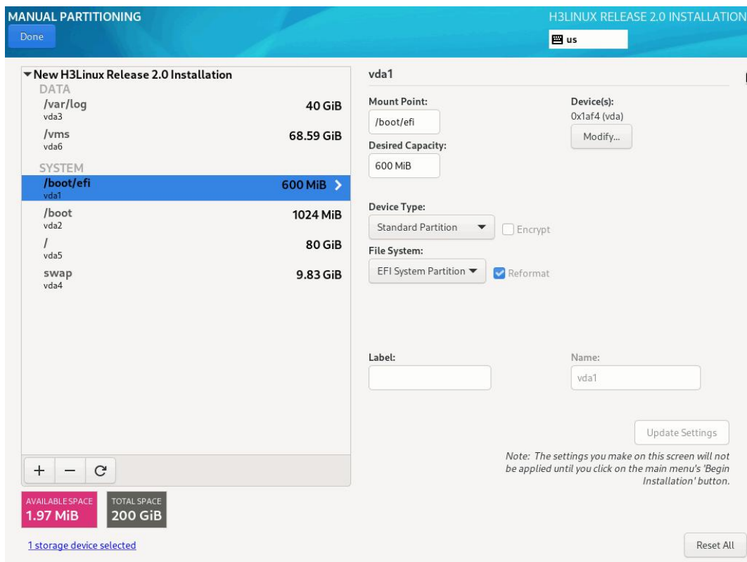
图 4-17 分区完成
