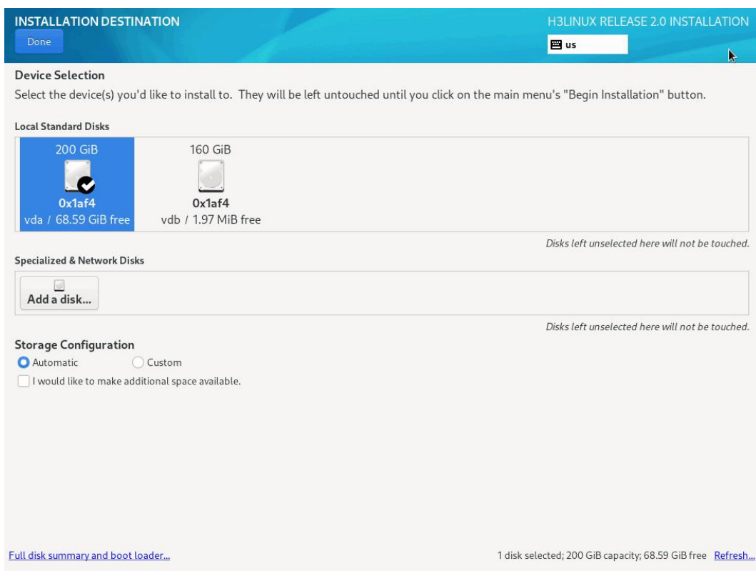
图 4-11 选择系统盘页面
