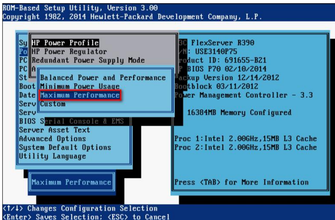
图 4-1 配置电源
