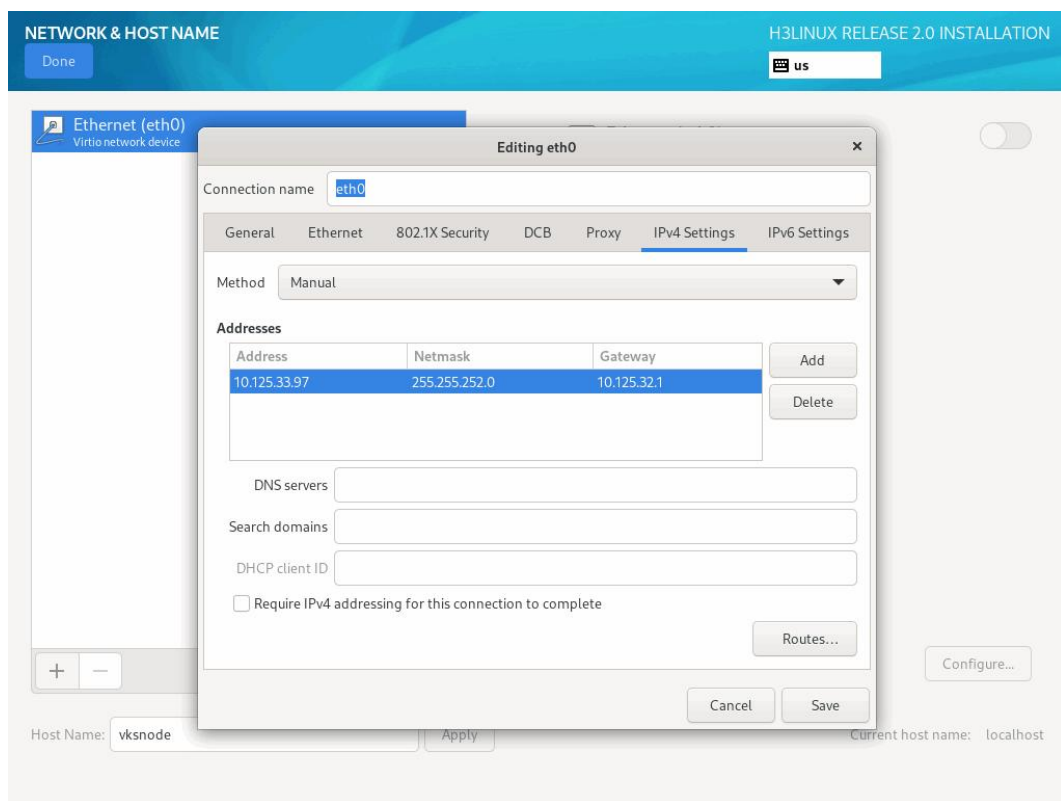
图 4-7 网络设置
