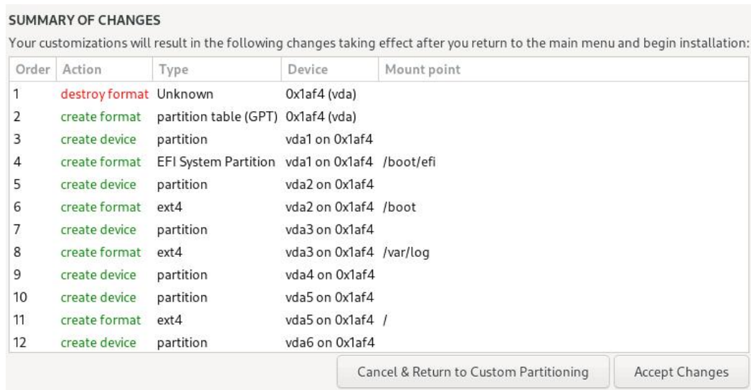
图 4-18 确认对话框
