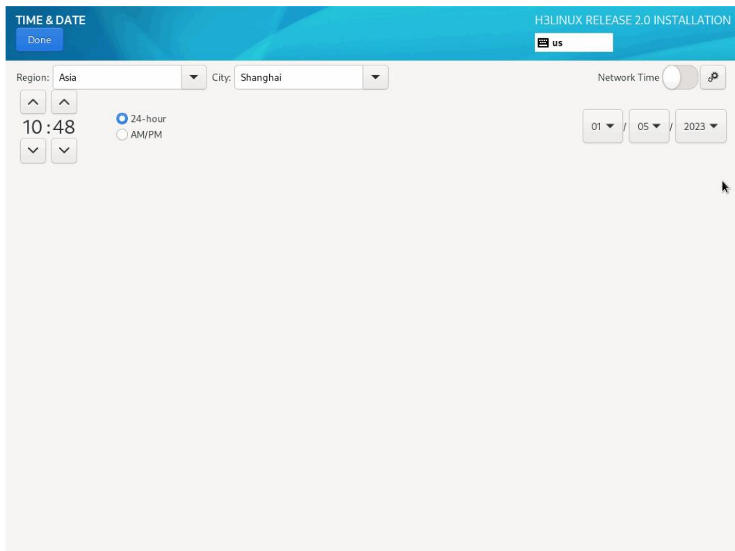
图 4-20 时区设置
