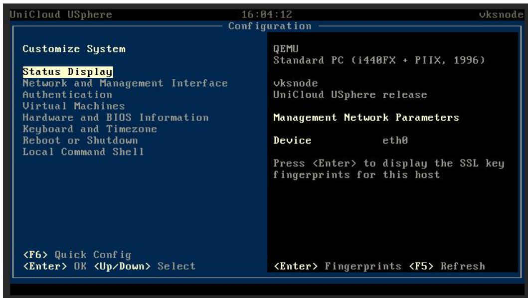
图 4-26 参数配置页面
