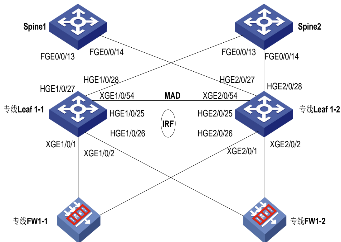
图A-9 专线 Leaf 组网图
